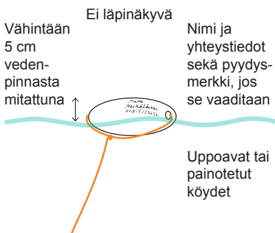
Kuva 2. Havainnekuva rapumerrassa käytettävästä kohosta.
