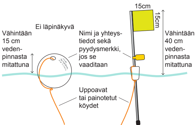
Kuva 4. Havainnekuva kohosta ja lipusta, joita käytetään pyydysen merkitsemiseen vesiliikennealueen ulkopuolella.
