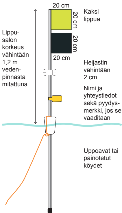
Kuva 3. Havainnekuva pyydyslipusta, jota käytetään pintapyydysen merkitsemiseen vesiliikennealueella.
