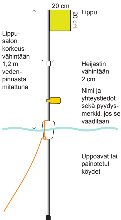
Kuva 1. Havainnekuva pyydyslipusta, jota käytetään pyydyn merkitsemiseen vesiliikennealueella.
